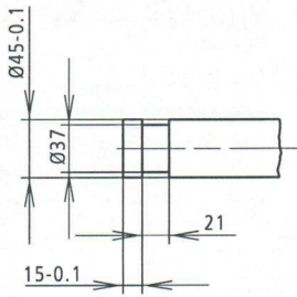
Auswerferbolzen
