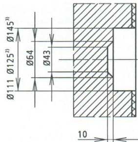
Maße für Duroplastwerkzeuge
