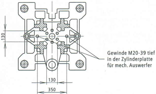
Ausdrehung im Werkzeug nur, wenn kurzer Anguss gewünscht wird
